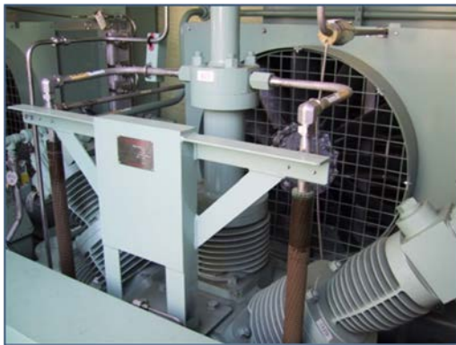
水素ガス圧縮機 (95MPa)
